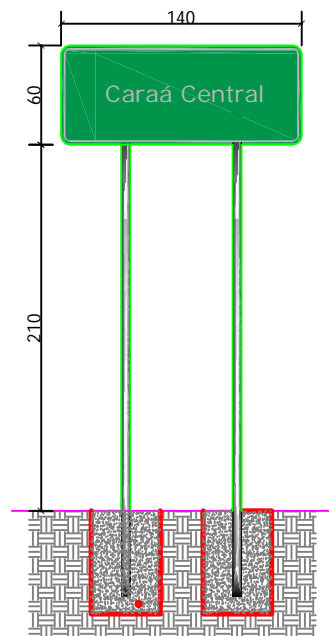
Base concretada - Dimensão da cava 40x40x60cm
