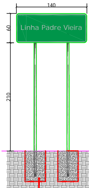
Base concretada - Dimensão da cava 40x40x60cm
